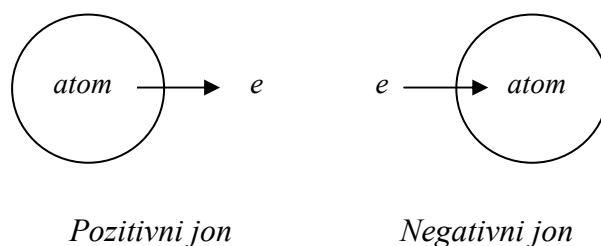
Slika 2-3 Jonizacija atoma
