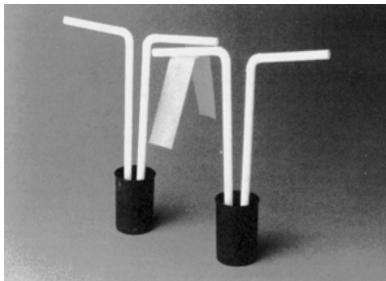
Slika 7-2 Elektroskop
