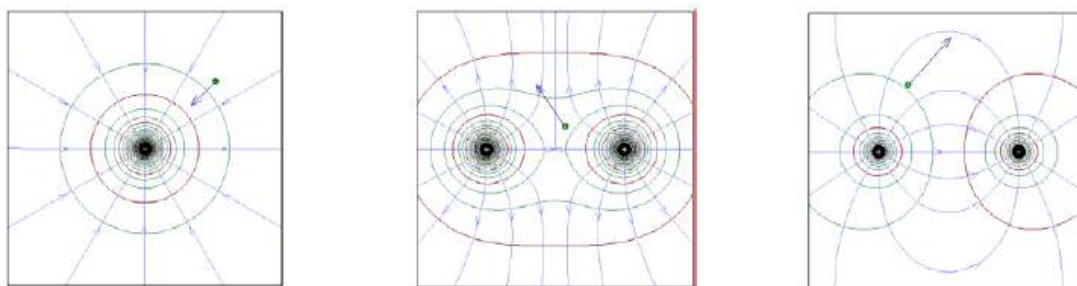
Slika 4-1 Ekvipotencijalne linije
