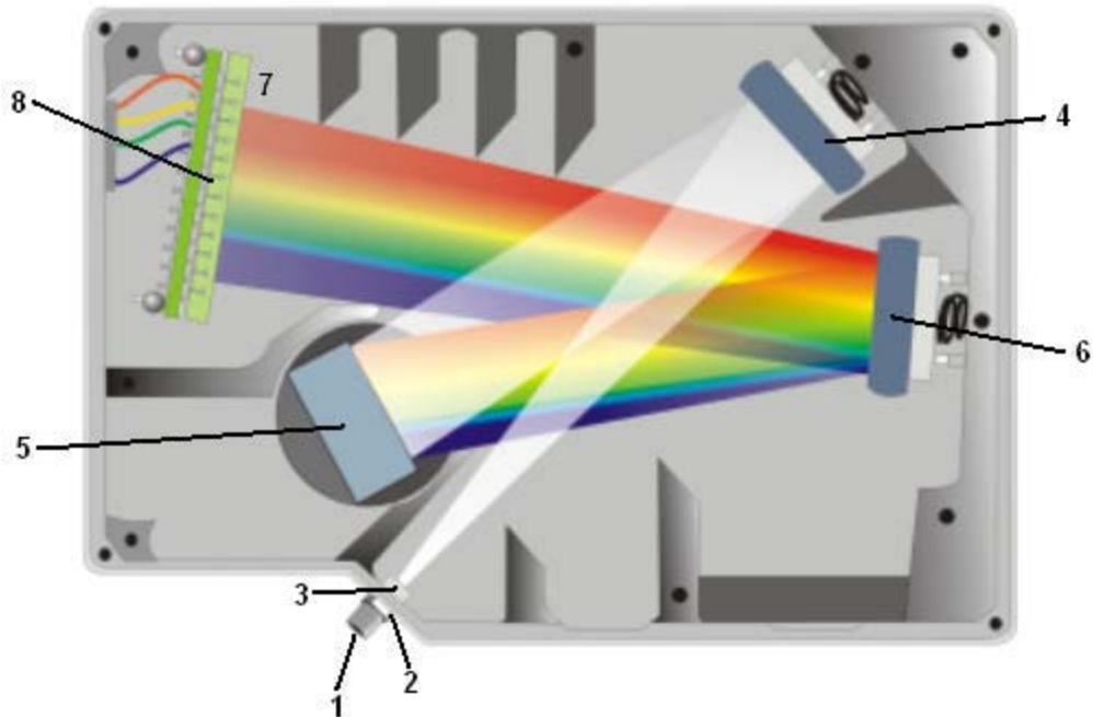
Slika 6.2. Optička šema spektrometra Oceans Optics HR2000
